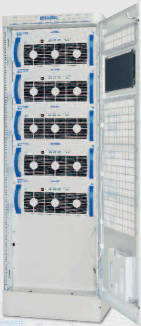
Fig. 4: ENERTRONIC modular SE, 200 kW
